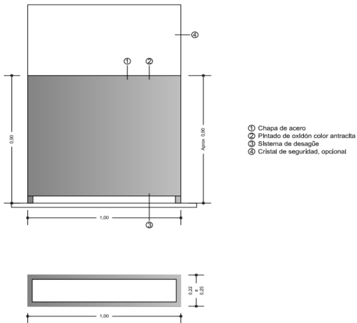
Detalle 2.- Elemento de protección en terrazas
