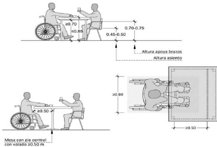
Detalle 1.- Dimensionado de mobiliario conforme a normativa
