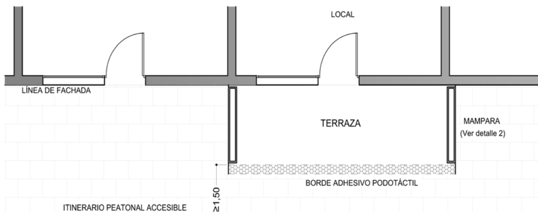
Figura 2.- Ubicación de terraza junto a línea de fachada
