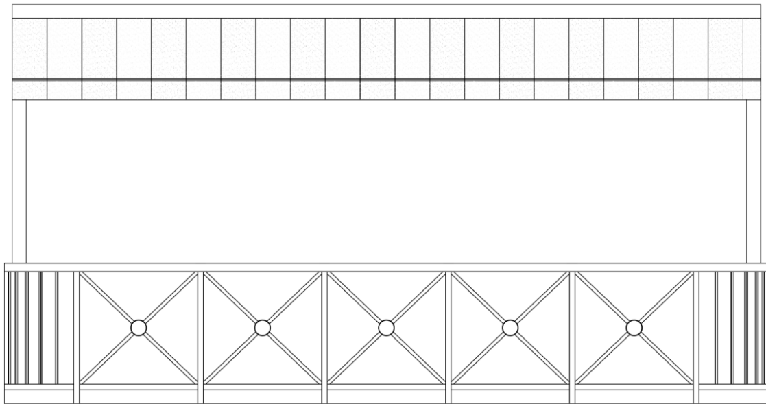
Vista frontal- Toldo
