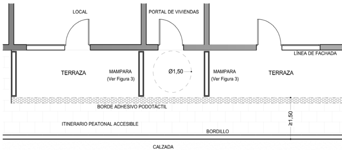
Figura 4.- Ubicación de terrazas en línea de fachada junto a portales de otros usos
