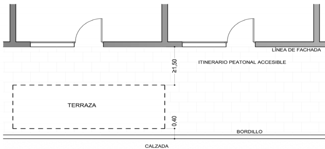
Figura 1.- Ubicación de terrazas sobre acera conforme normativa de aplicación
