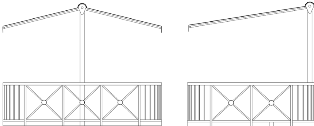
Vistas laterales- Toldo simple/ duplo
